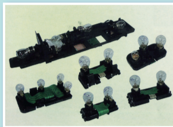
Плата фонаря для автомобилей BA3 2108-3716096/097, 2110-3716096/097, 2111-3716096/097, 21213-3716096/097
